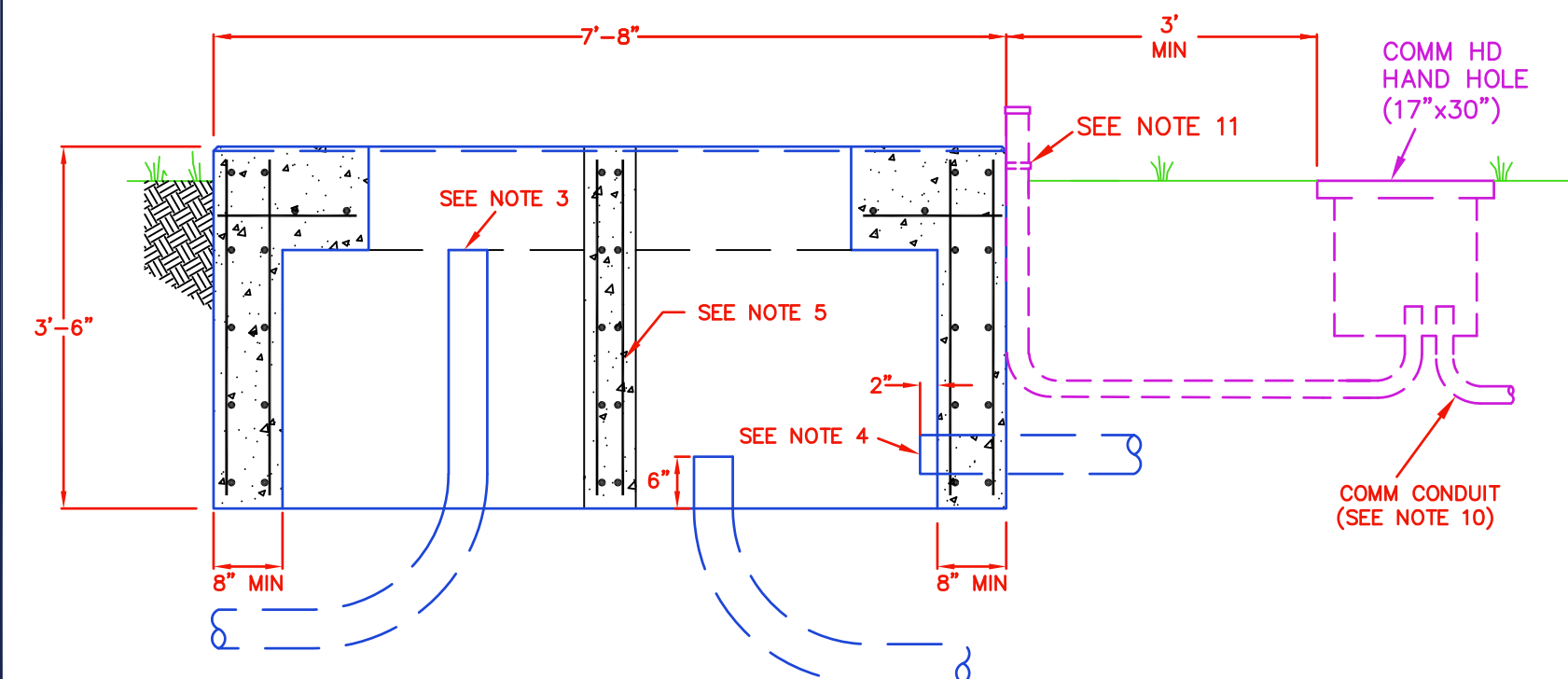
SECTION A-A
