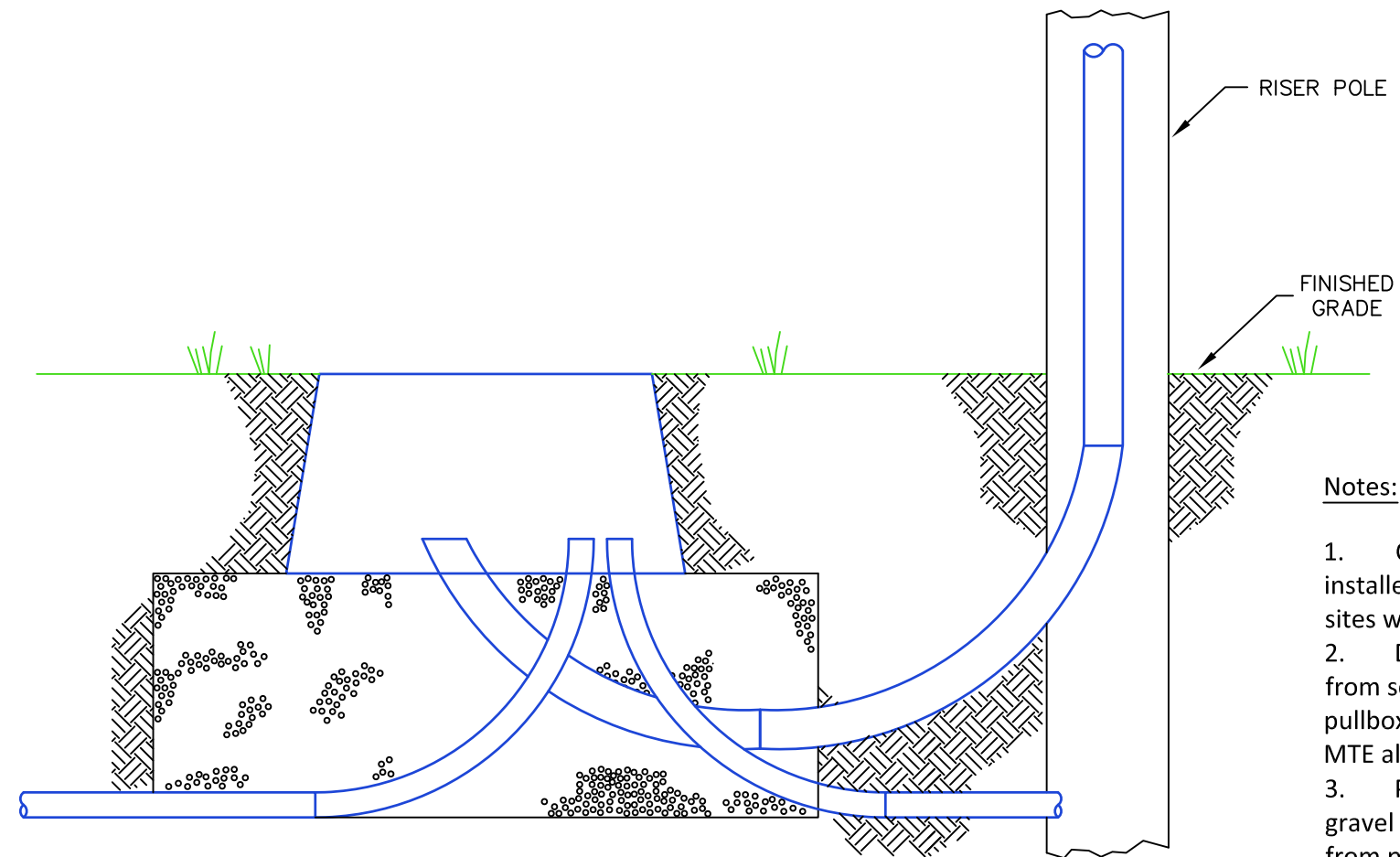
SIDE VIEW SCALE: NONE
